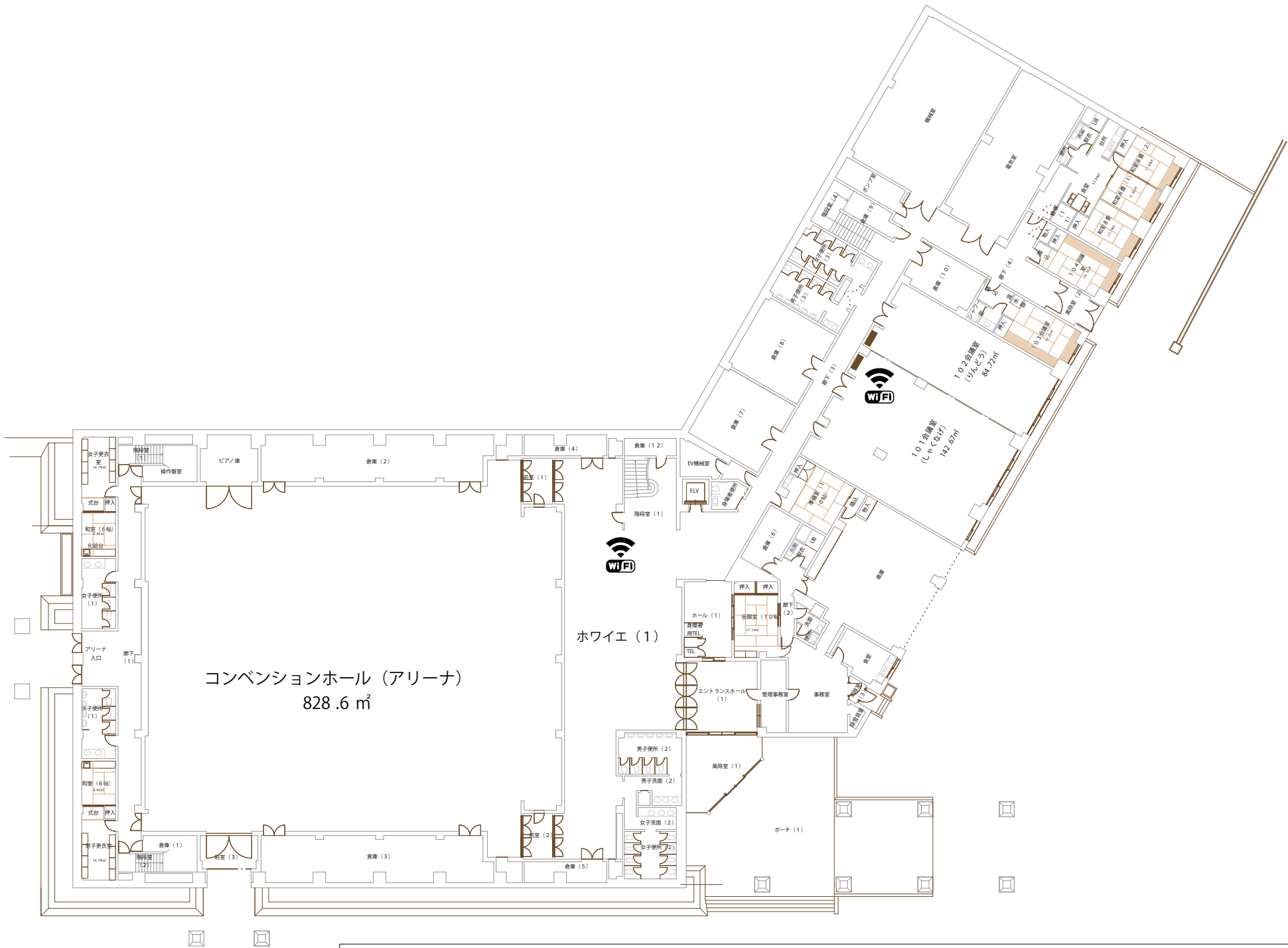
98 総合会館 1階平面図 縮尺1/400 印刷サイズ A4
