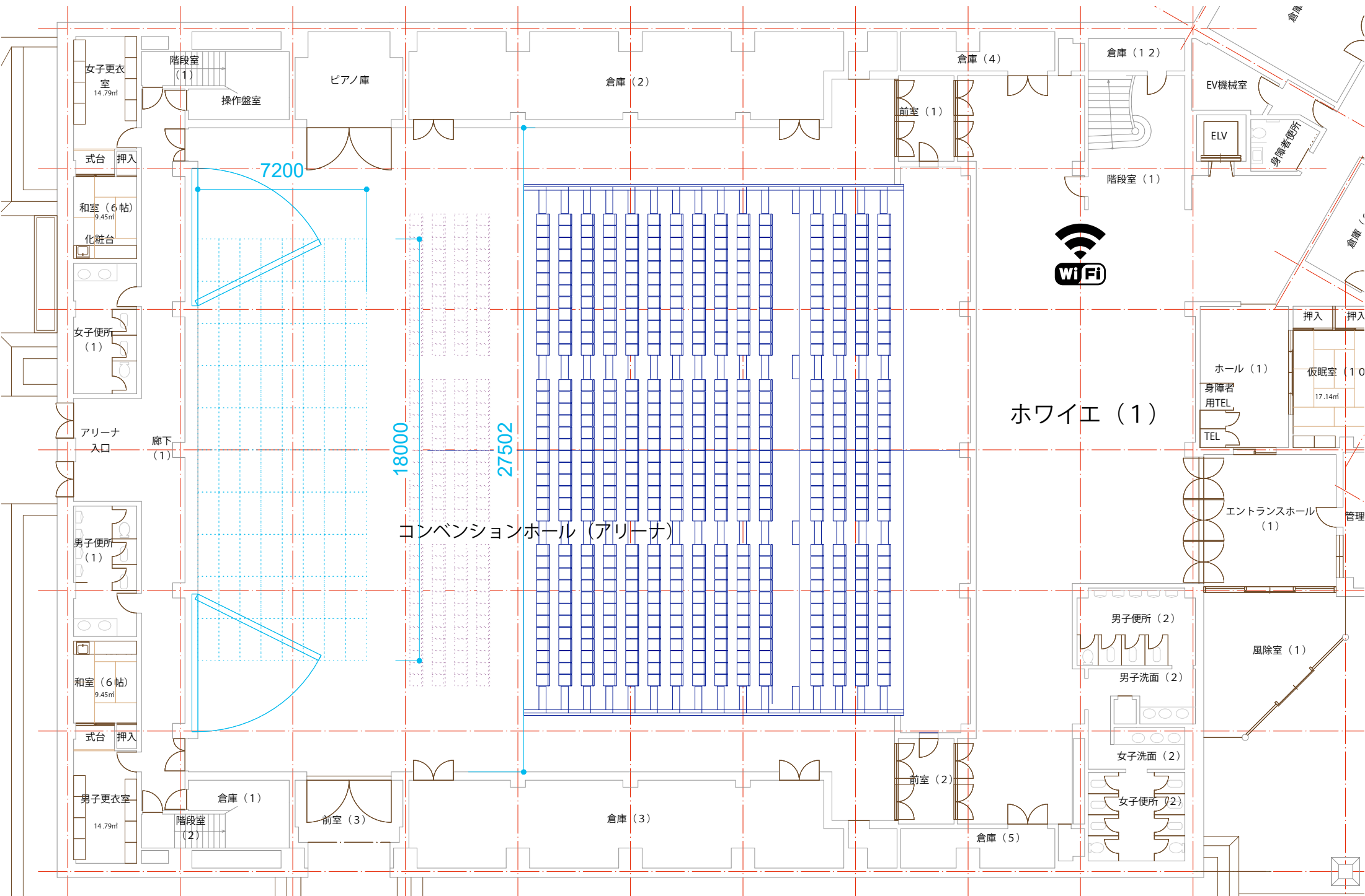
98ホール 1階 平面図 (通常ステージ：通常仕様) 縮尺 1/200 印刷サイズ A4
